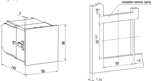
Рисунок 2 – Габаритные размеры корпуса Щ4
