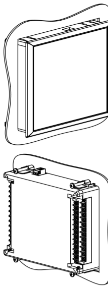
Рисунок 4 – Монтаж прибора щитового крепления
