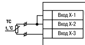
Рисунок 8 – Двухпроводная схема подключения ТС
