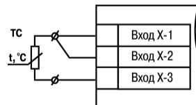
Рисунок 7 – Трехпроводная схема подключения ТС
