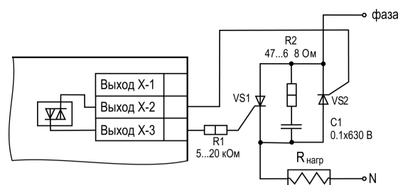
Рисунок 16 – Схема встречно-параллельного подключения двух тиристор к ВУ типа С RC-фильтры предназначены для защиты элементов схемы от перепадов напряжения в сети.
