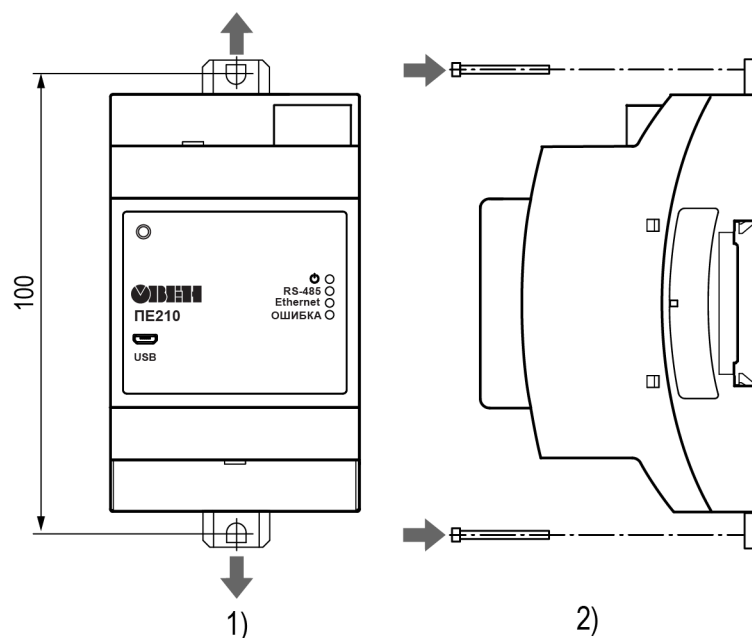
Рисунок 4.2 – Крепление винтами
