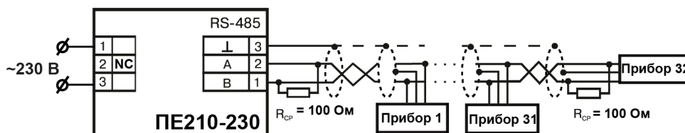
Рисунок 5.2 – Схема подключения PE210 с номинальным напряжением питания 230 В переменного тока
