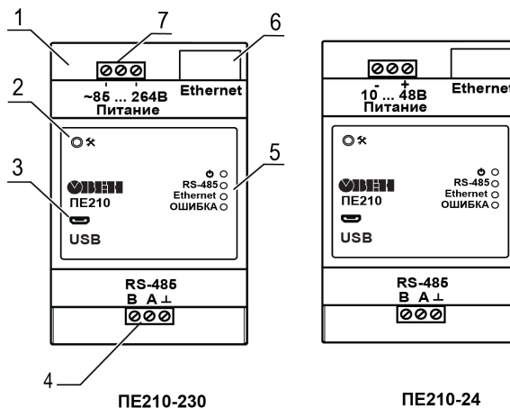
Рисунок 6.1 – Общий вид прибора
