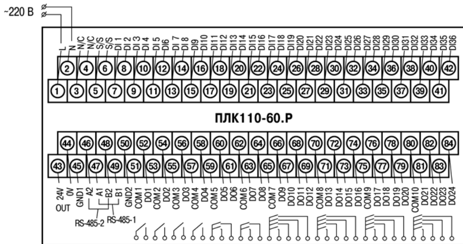
Рисунок Б.1 – Схема расположения и назначение клемм на ПЛК110-240.60.P. Схема для ПЛК110-24.60.P– аналогична, полярность при подключении клемм питания аналогична рисунку Б.2
