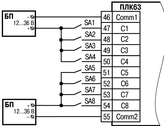
Рисунок Б.1 – Подключение датчиков к дискретным входам
