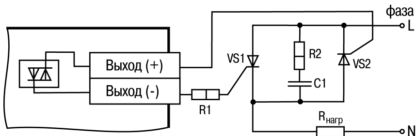
Рисунок Б.12 – Схема подключения нагрузки к ВЭ типа «С» двух тиристоры, подключенных встречно-параллельно ( R_2=47\dots 68 \text{ Ом} , C_1=0.1\text{мкф}\times 630 \text{ В} )
