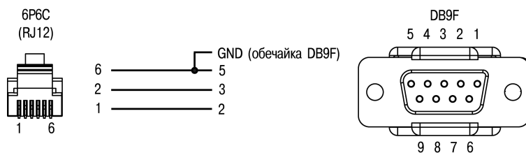
Рисунок В.2 – Схема кабеля КС2
