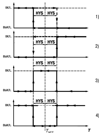
Рисунок 7.9 – Типы логики работы регулятора
