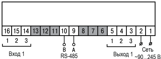
Рисунок 5.3 – Общая схема подключения TPM201-H2
