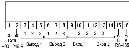
Рисунок 5.2 – Назначение контактов клеммника TPM202-H, -Щ1 и -Щ2
