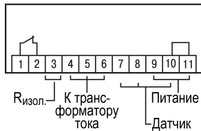
Рисунок 5.2 – Назначение контактов клеммника
