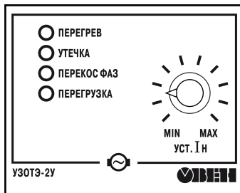
Рисунок 6.2 – Лицевая панель прибора
